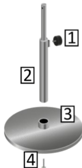
Bodenständer montieren
